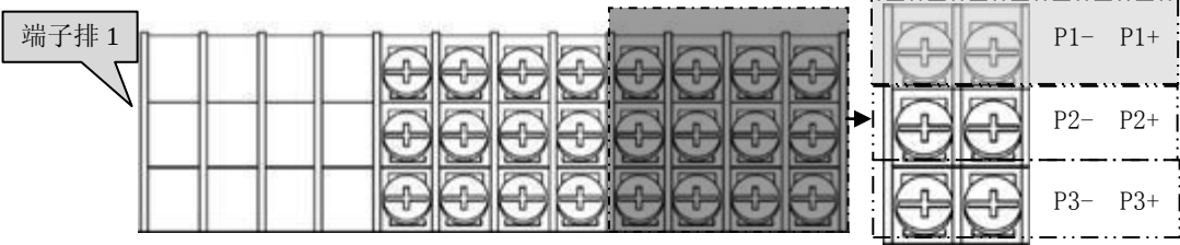
注：连接如上，共 12 组输出端子。图 2-2-3-D
