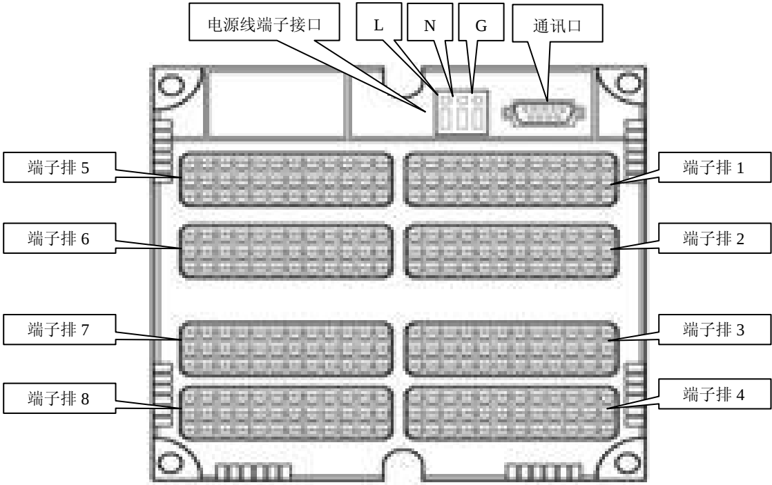
图 2-2-3-A 端子排列图
