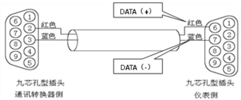
图 2-2-8 485 通讯联网示意图
