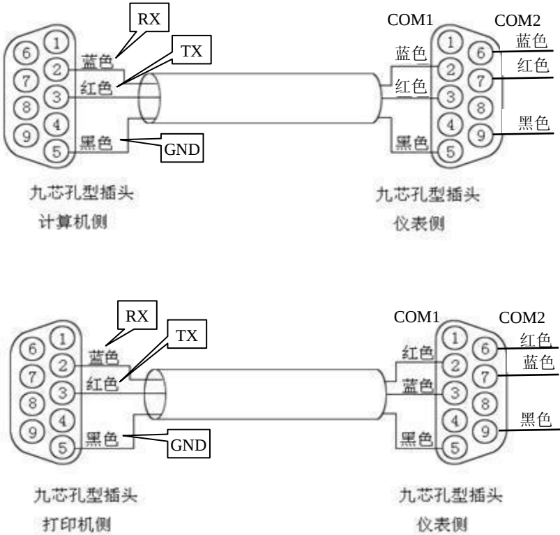
图 2-2-7-B 打印机与仪表间的 RS-232C 通讯线
