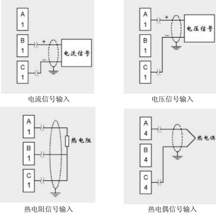
图 2-2-4 模拟量输入信号接线图
