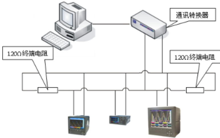
图 2-2-7 485 通讯联网示意图
