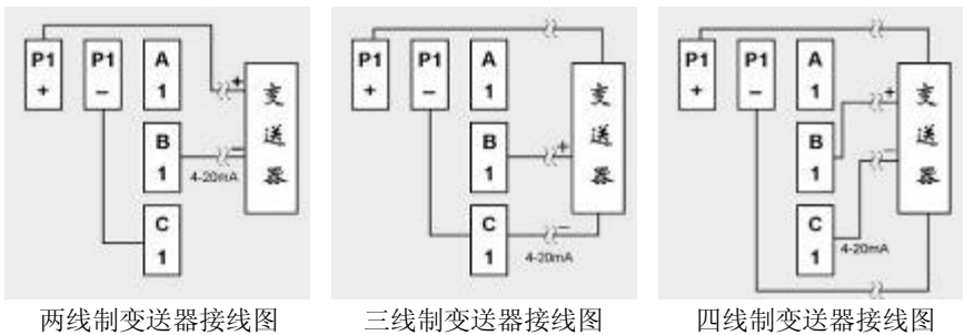
图 2-2-5 带馈电变送器接线图
