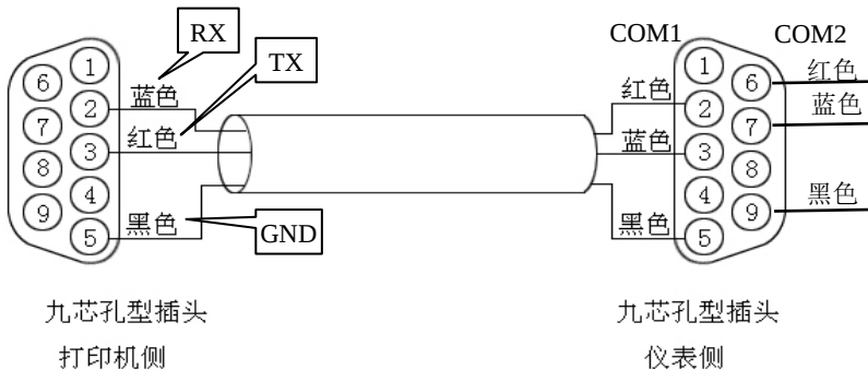
图 2-2-7-B 打印机与仪表间的 RS-232C 通讯线
