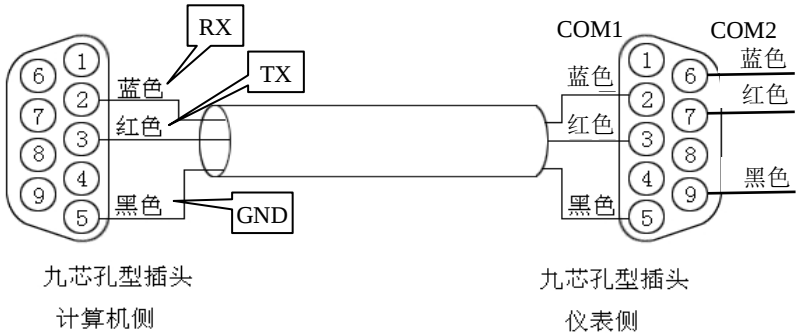
图 2-2-7-A 计算机与仪表间的 RS-232C 通讯线
