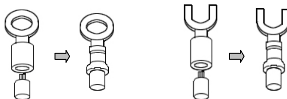
用绝缘套筒压接线端子（4mm 螺钉用）
