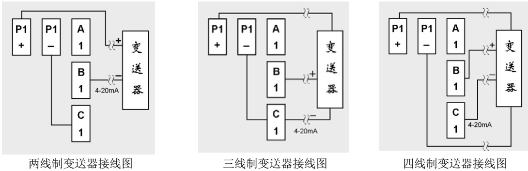
图 2-2-6 带馈电变送器接线图
