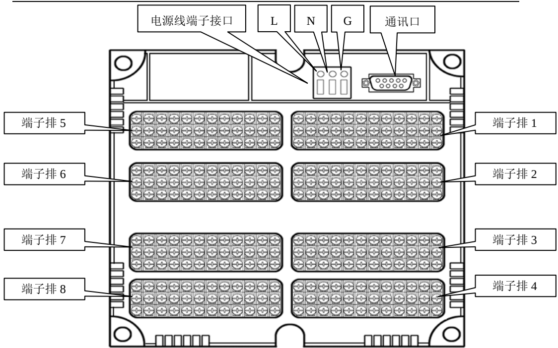
图 2-2-3-A 端子排列图
