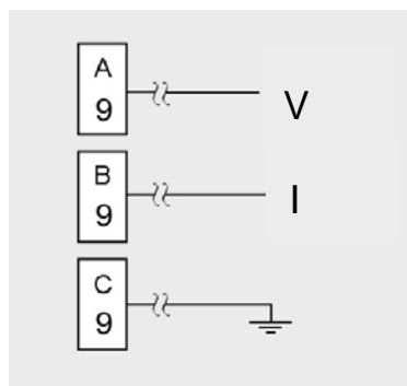
变送输出
