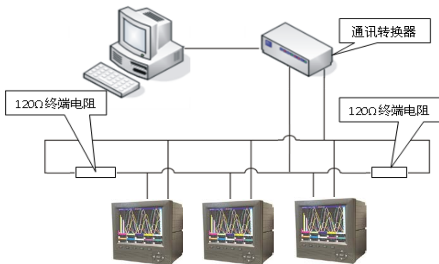
图 2-2-8 485 通讯联网示意图
