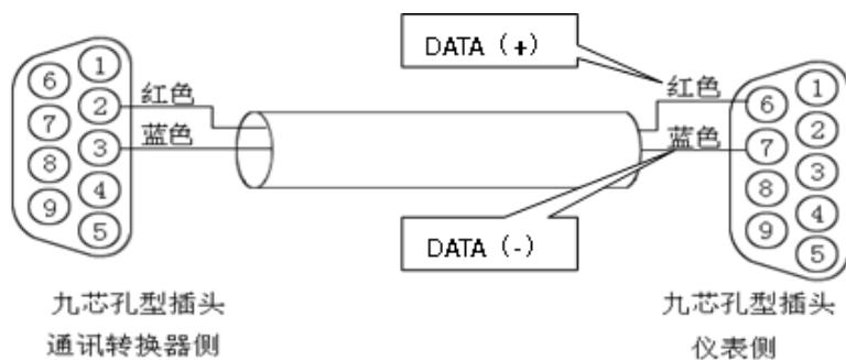
图 2-2-8 485 通讯联网示意图
